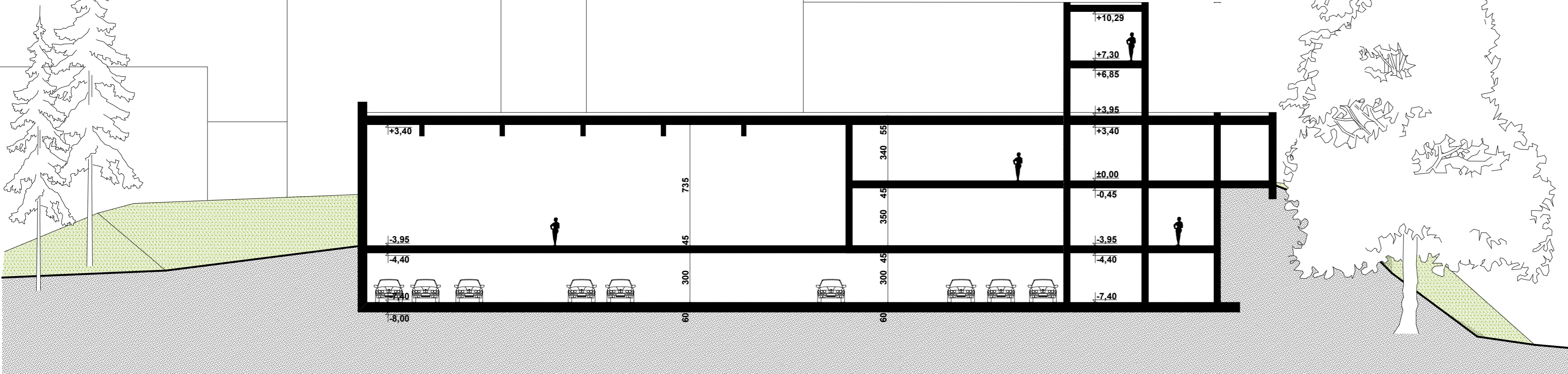
Przekrój A-A
